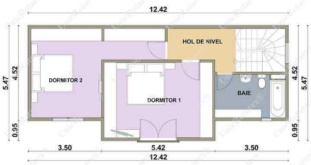
PLAN ETAJ
